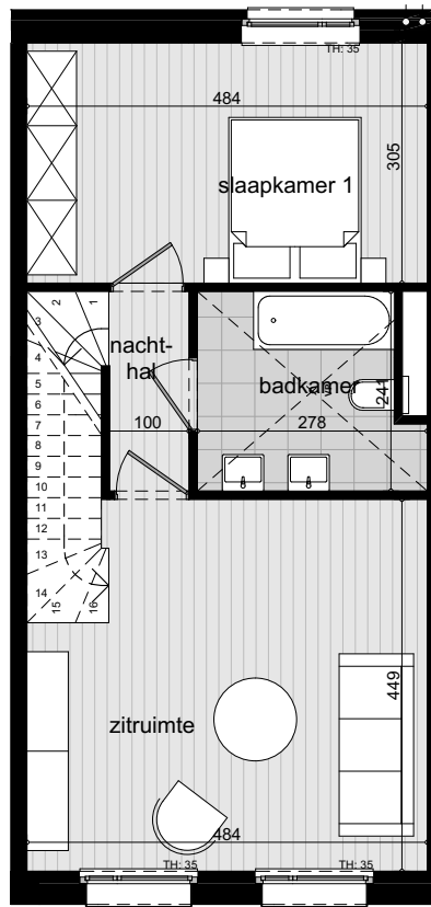
verdieping +01
