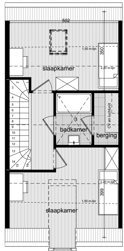
verdieping +02
