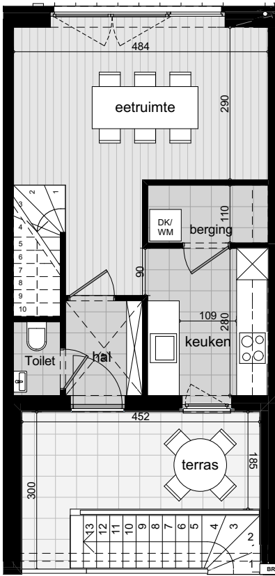
gelijkvloers
