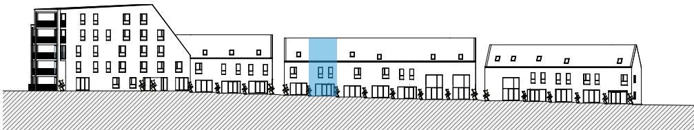
BLOK A - ACHTERGEVEL - NOORD
