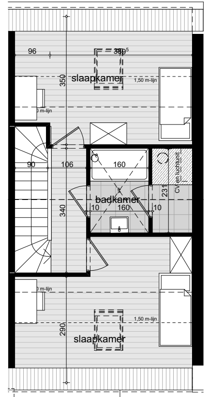
verdieping +02
