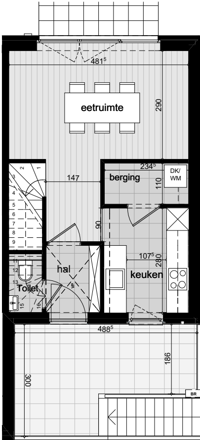
gelijkvloers
